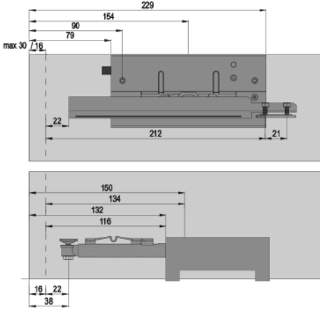
Dış kapak için mekanizma montaj ölçüleri
