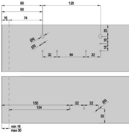
Dış kapak için mekanizma montaj ölçüleri
