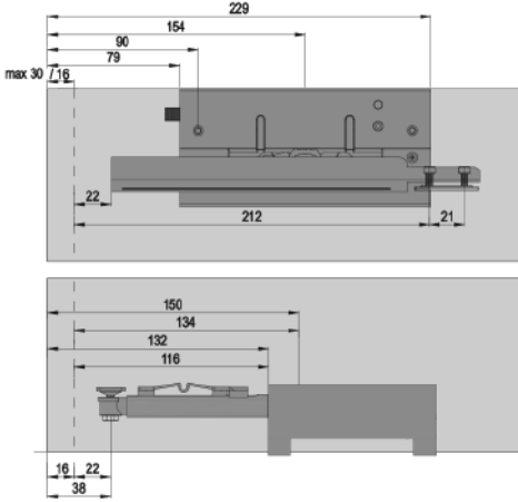
İç kapak için mekanizma montaj ölçüleri
